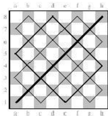
Рисунок 2. Шашечная доска с прорисованными диагоналями (русские шашки).
